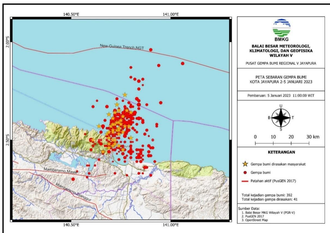
Gambar 2.10. Titik Gempa Periode 02 Januari s/d 05 Januari 2023
